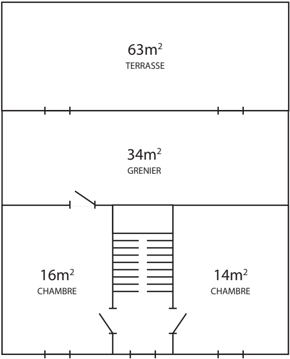
2ème étage
